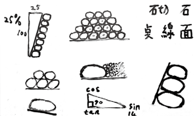
▲ 砌石護坡手繪圖
