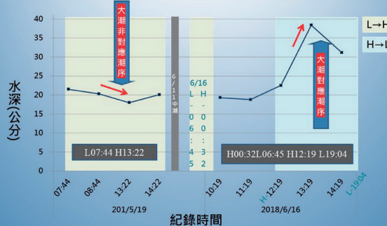
社子島四斑細蟪樣線水位變化-大潮
