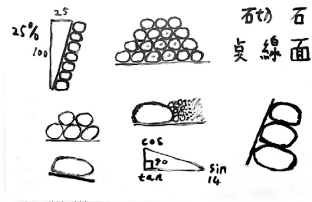
▲ 砌石護坡手繪圖
